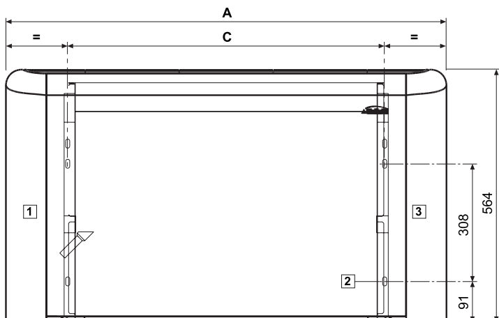
Méretek mm-ben
