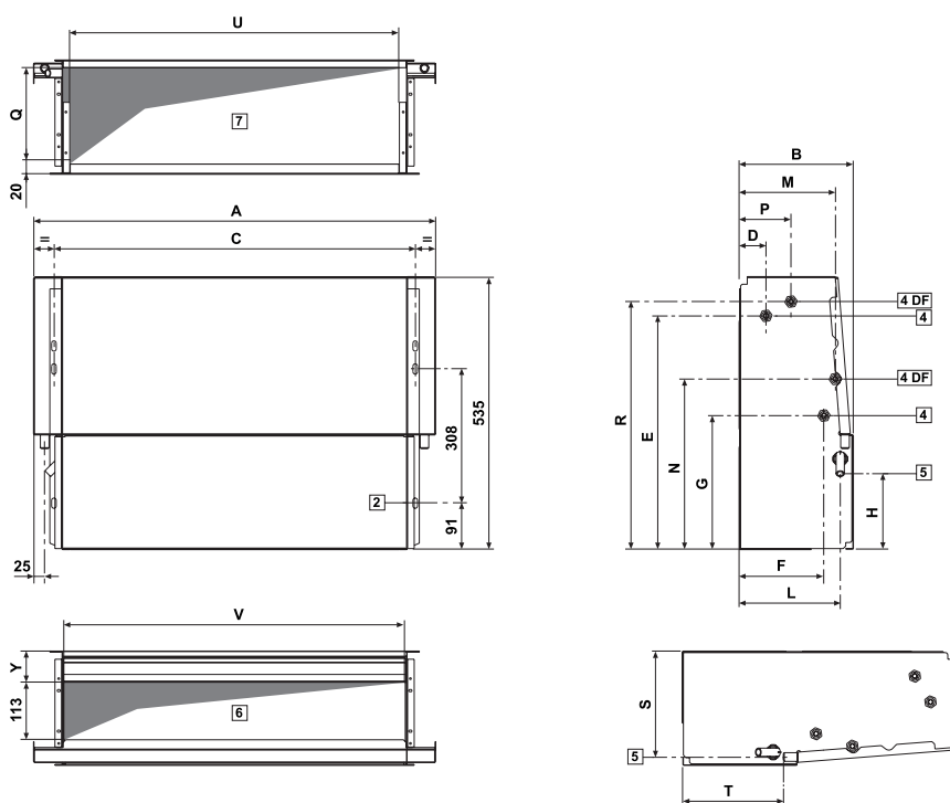
Méretetek mm-ben
