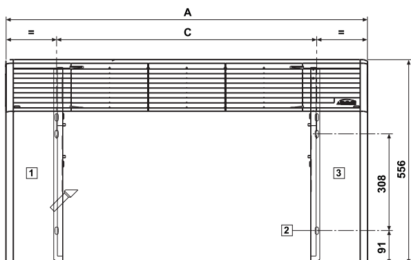
Méretek mm-ben
